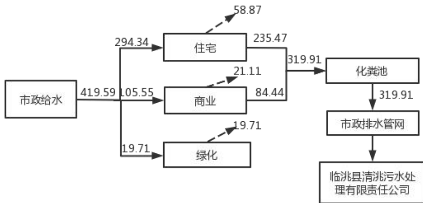
图 2-1 项目水平衡示意图 单位：m 3 /d
